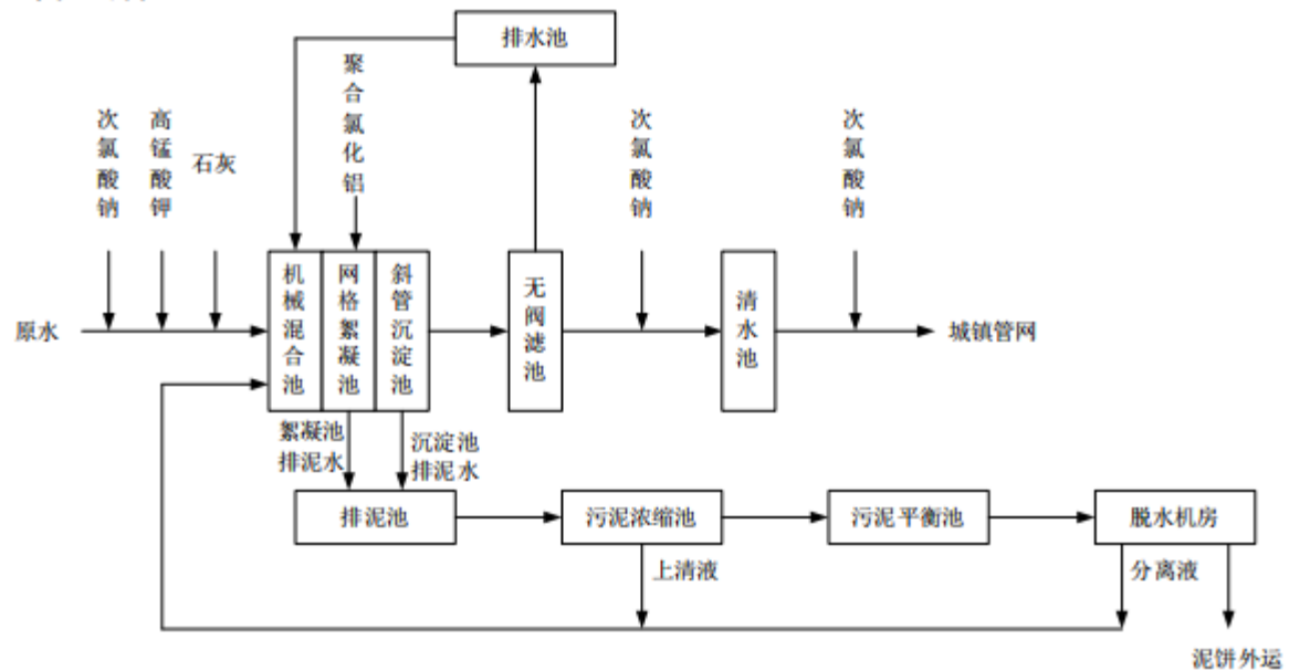
图 2-3 水厂营运期工艺流程及产污环节图
